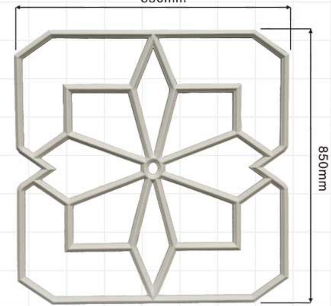
M-7411 D:850x850x20mm
