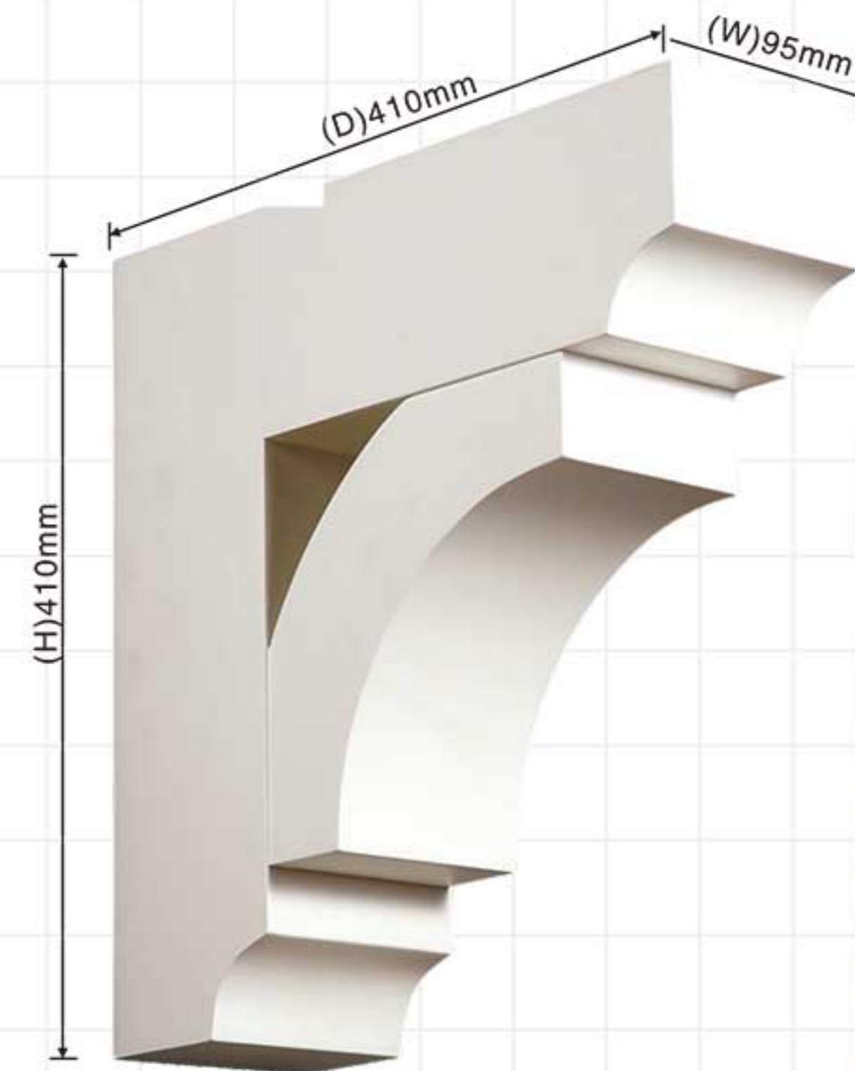
GL-6045 (H)410x(W)95x(D)410mm
